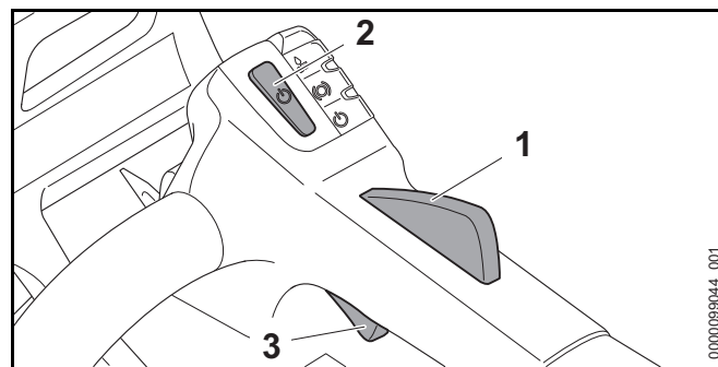
Bloqueo del gatillo (1), botón de retención (2) y gatillo (3)
